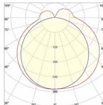
Lichtverdeling
