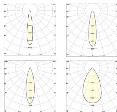
Lichtverteilung
