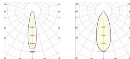
Lichtverteilung
