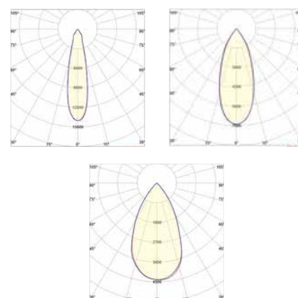
Lichtverteilung
