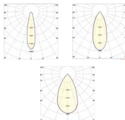
Lichtverteilung
