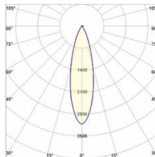
Lichtverteilung
