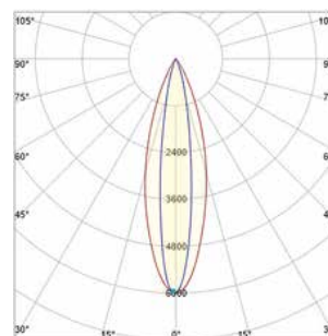
Lichtverteilung
