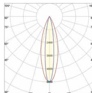
Lichtverdeling
