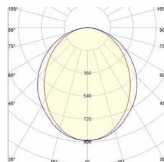
Lichtverteilung
