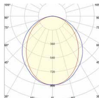
Lichtverteilung
